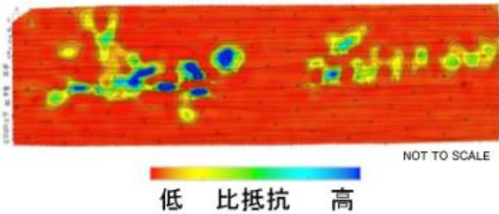
3次元逆解析結果 海底下45m 平面
